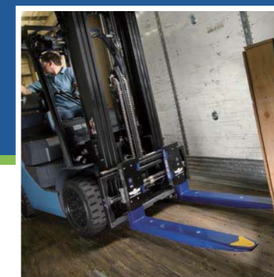
智能称重货叉 iForks
